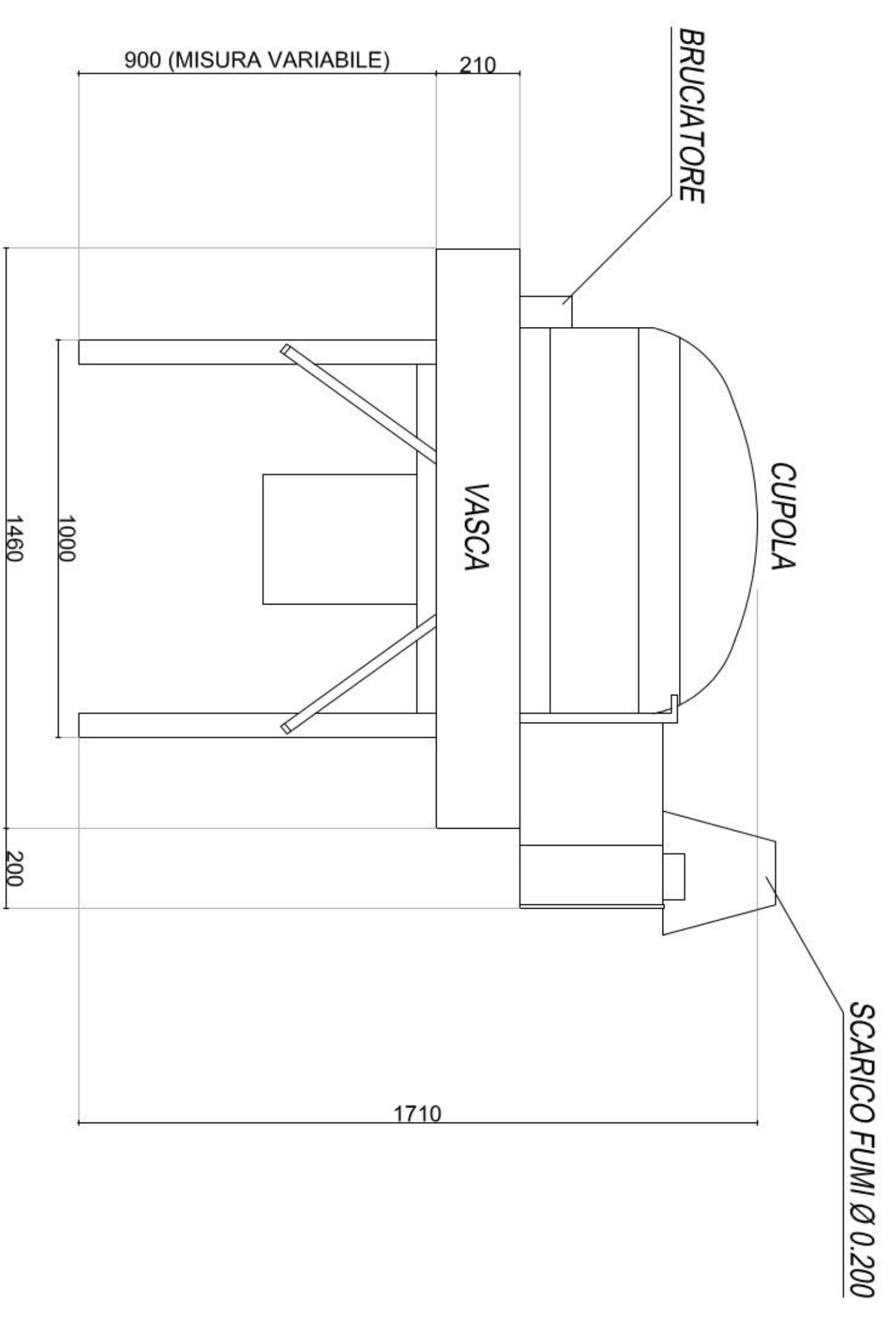
VISTA LATERALE FORNO 105 ROTOGAS SCALA 1:20
