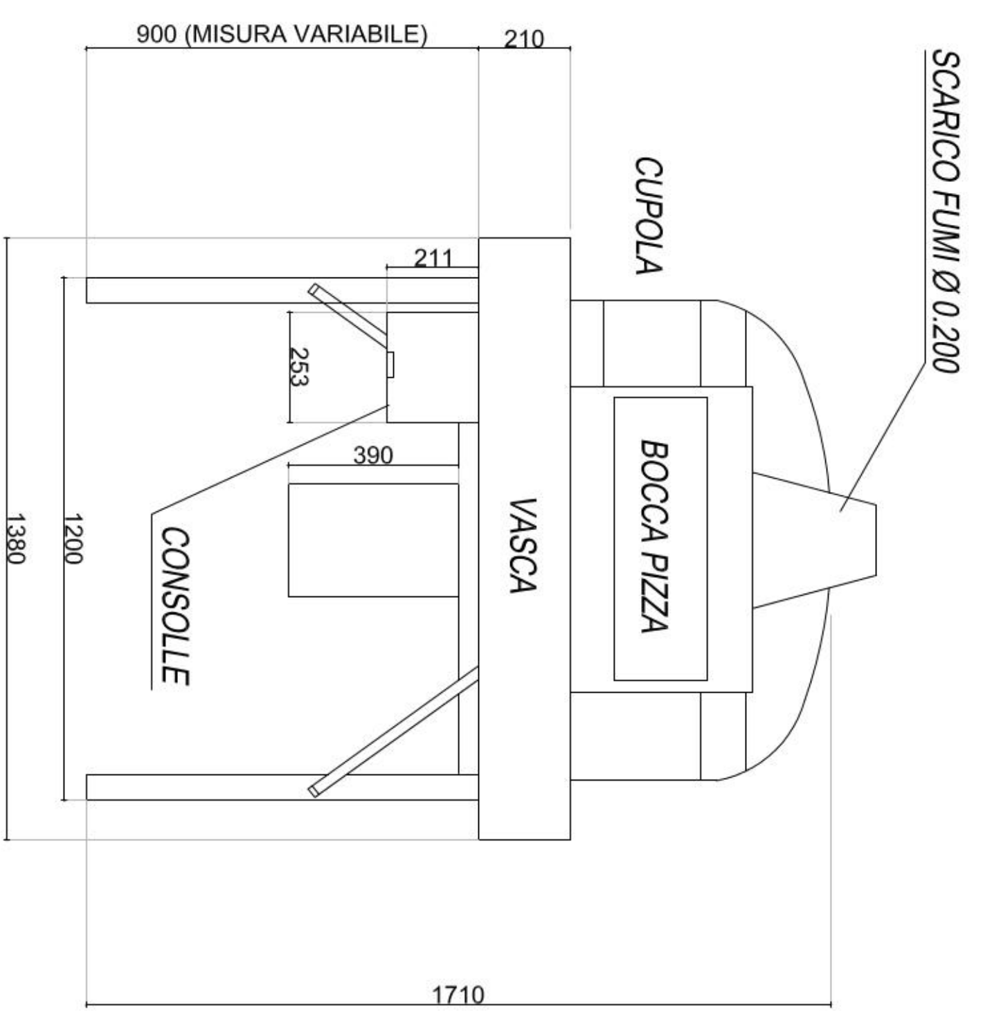
VISTA FRONTALE FORNO 105 ROTOGAS SCALA 1:20
